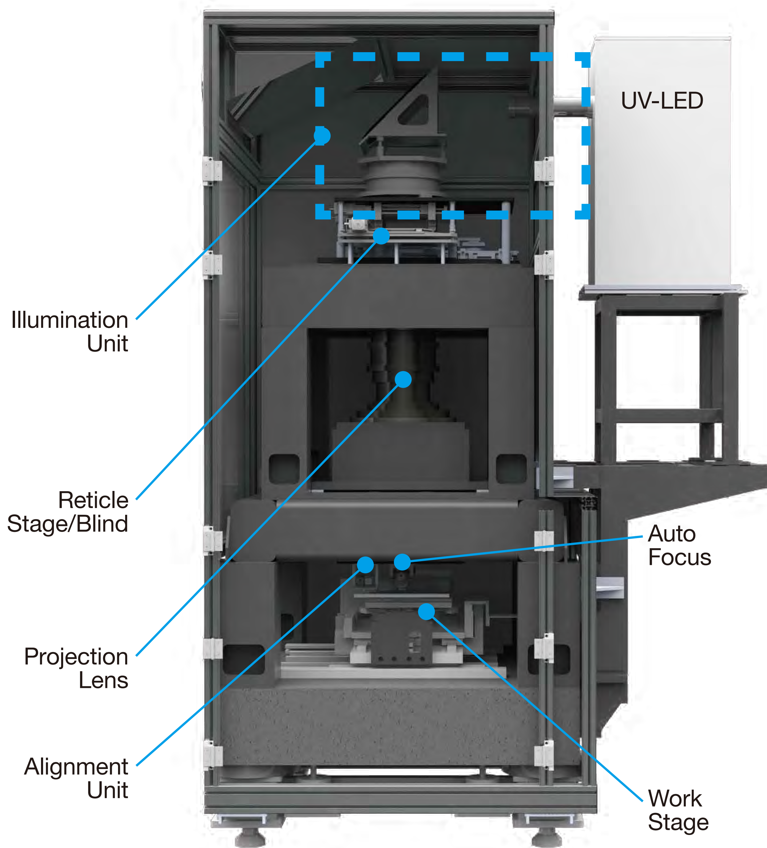
MRS1450 内部構成
